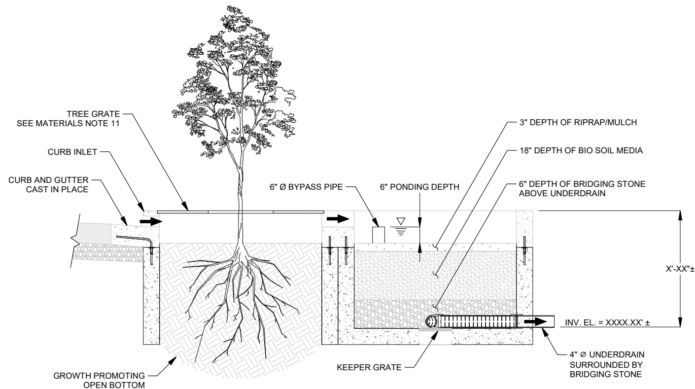
SECTION A-A
