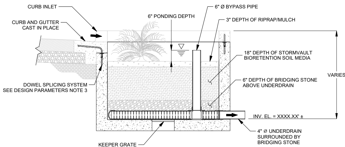
SECTION A-A
