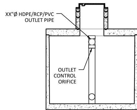
SECTION B-B SCALE: 1" = 60"
