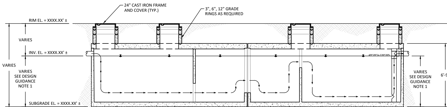
SECTION A-A SCALE: 1" = 60"
