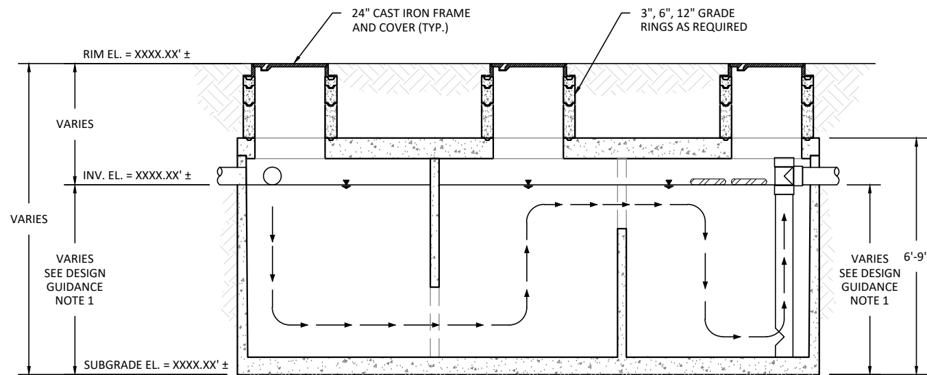
SECTION A-A SCALE: 1" = 45"
