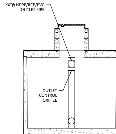
SECTION B-B SCALE: 1" = 45'
