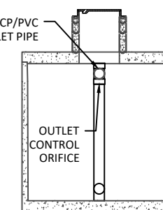
SECTION B-B SCALE: 1" = 75"
