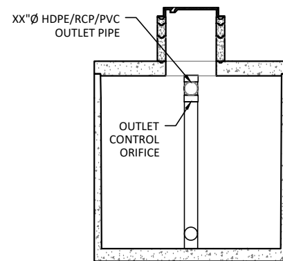
SECTION B-B SCALE: 1" = 60"
