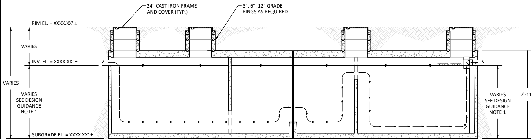
SECTION A-A SCALE: 1" = 60"
