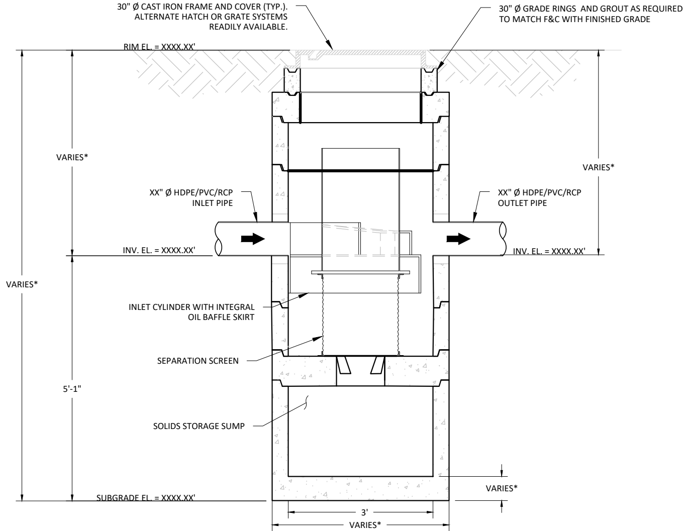
SECTION A-A SCALE= 1:30
