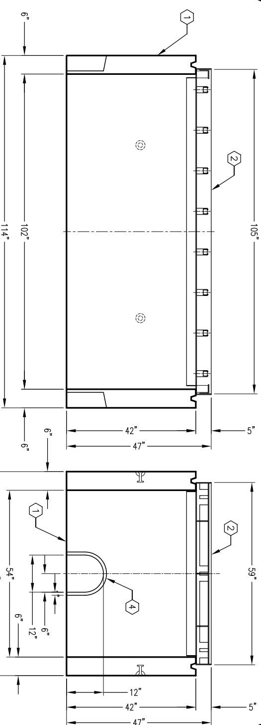
SECTION A-A
