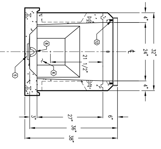
SECTION D-D
