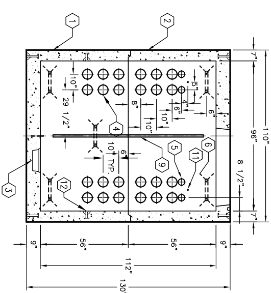
SECTION D-D
