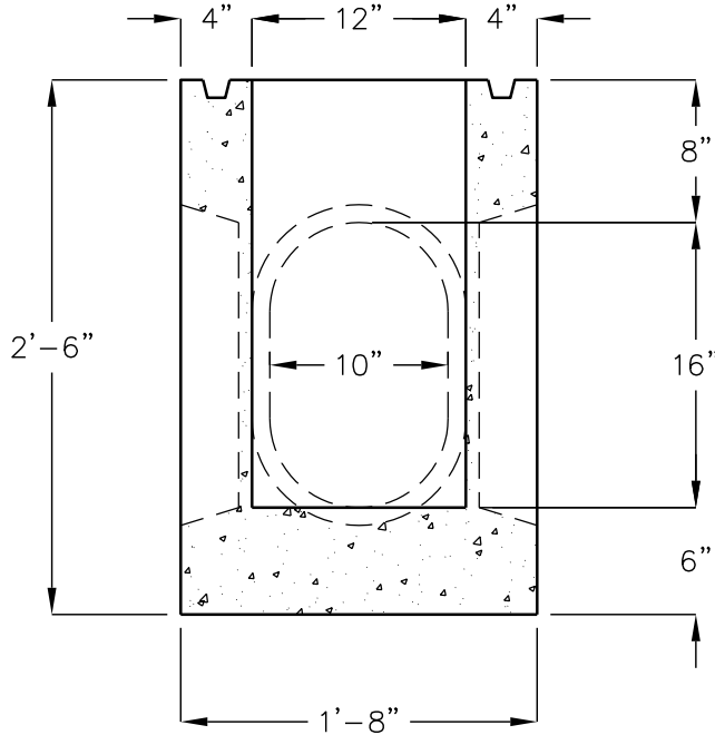
1212 D.I. BOX
