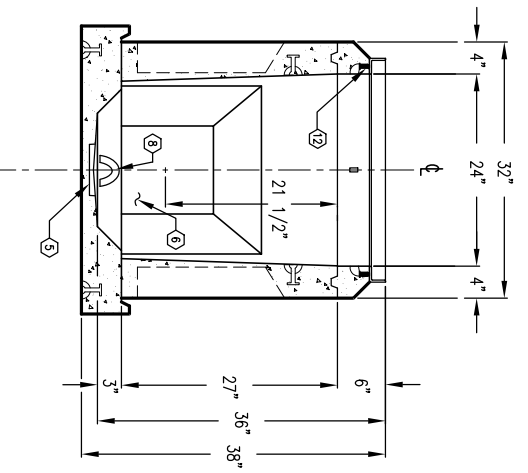
SECTION D-D
